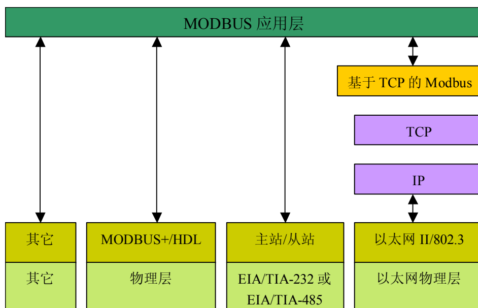
图 1：MODBUS 通信栈
