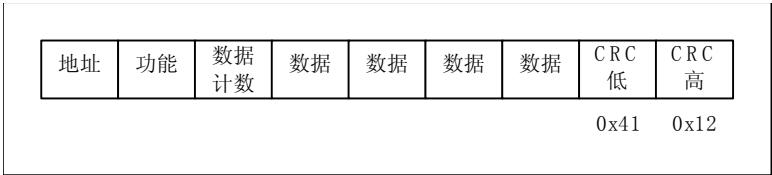
图 19: CRC 字节序列
