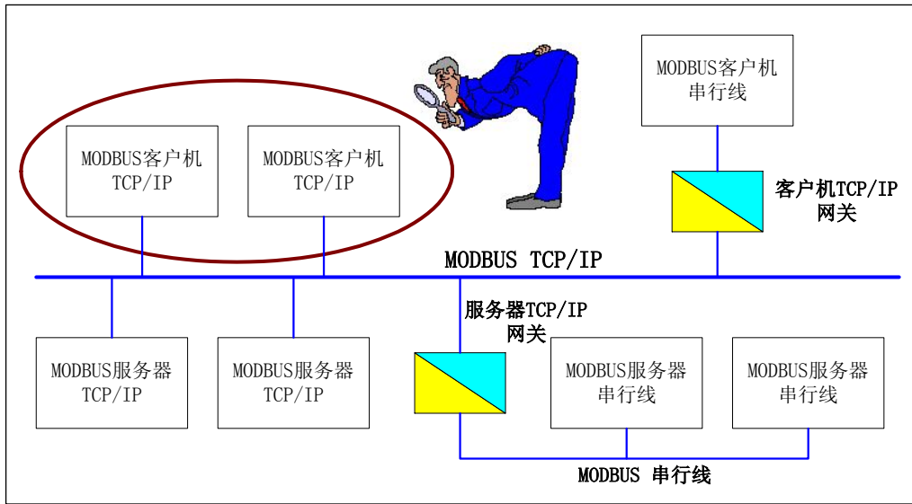
图 10: MODBUS 客户端
