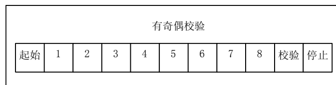
图 9: RTU 模式位序列
