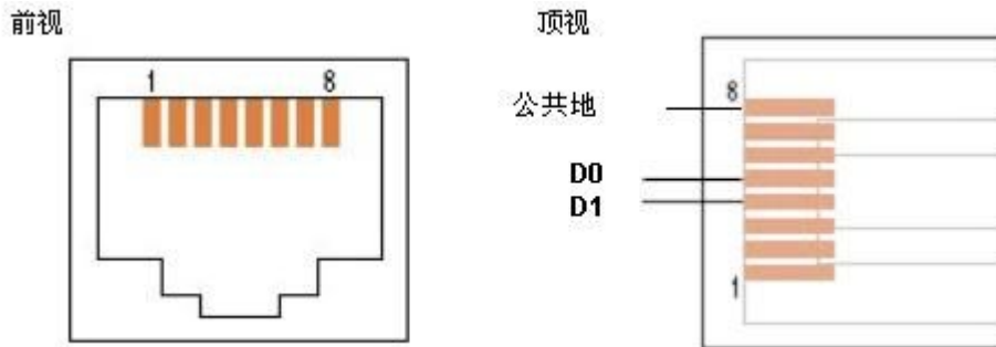
设备端 – 母连接器
