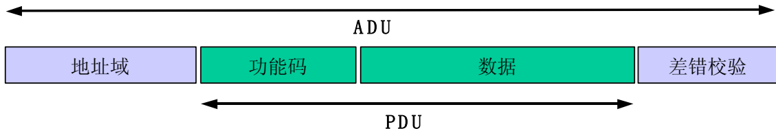
图 3: 通用 MODBUS 帧
