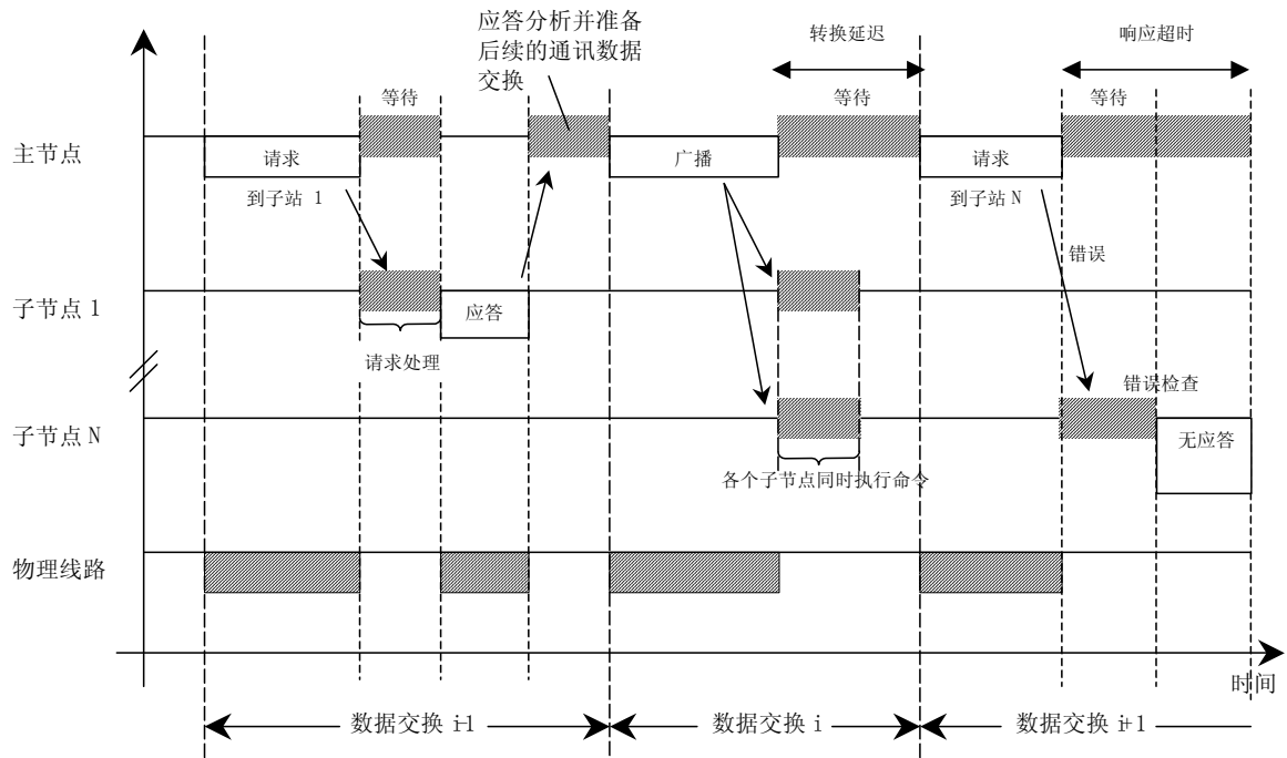
图 8: 各种情形的主/从通信时序图
