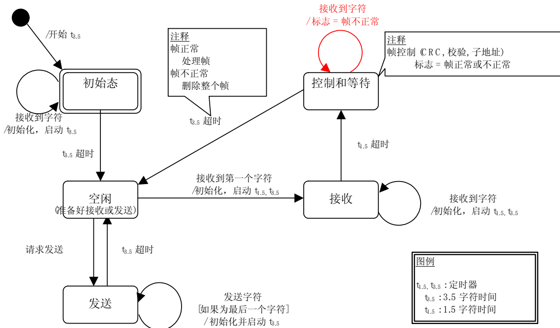
图 13: RTU 传输模式状态图
