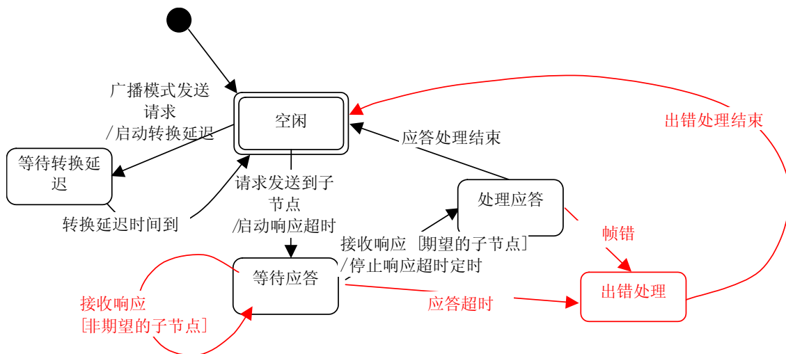
图 6: 主节点状态图
