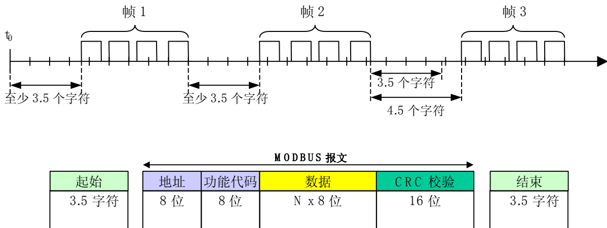
图 12: RTU 报文帧
