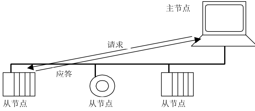
图 2: 单播模式
