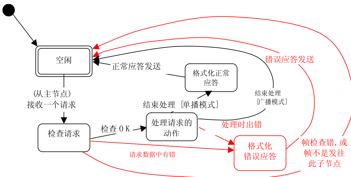
图 7: 子节点状态图
