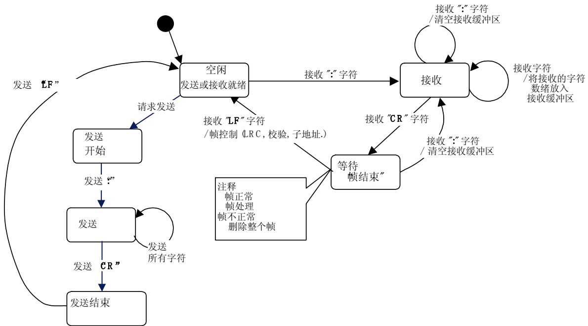
图 17: ASCII 传输模式状态图
