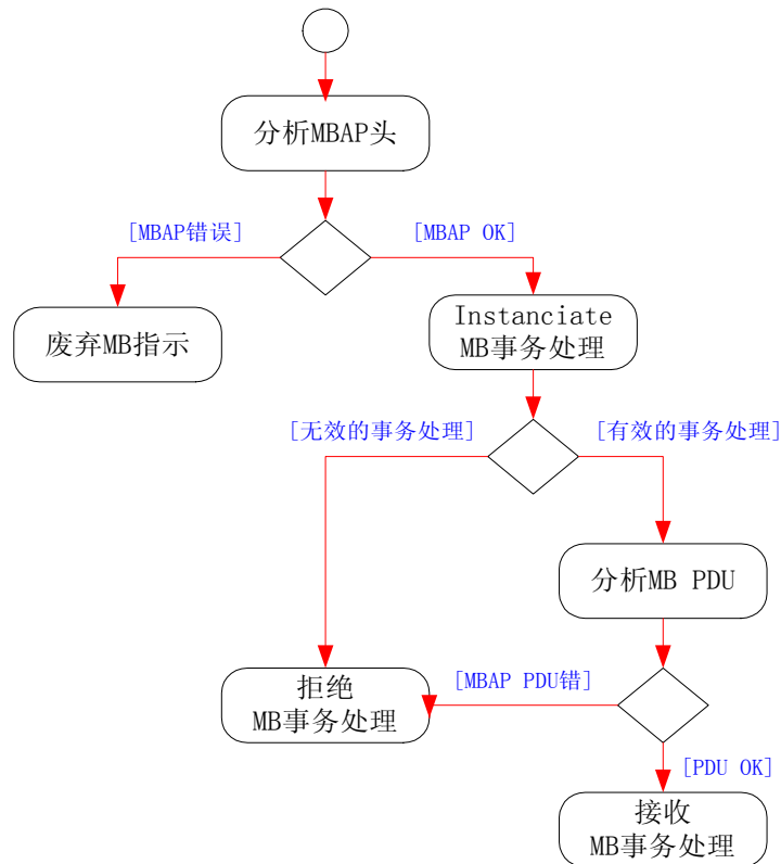
图 16：MODBUS PDU 检验操作流程图
